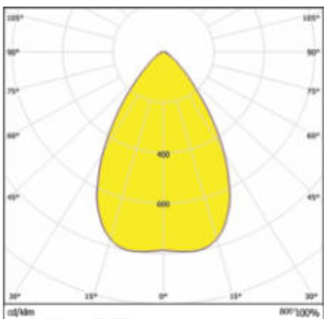
BO136-Aura-5050-60°(4 Rings)
