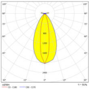
BO202-Sunbeam-1x1-3535-15x45°
