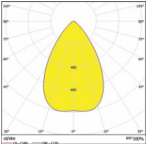
BO134-Aura-5050-60°(3 Rings)
