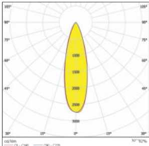
BO38-Sunbeam-1x1-3030-25°
