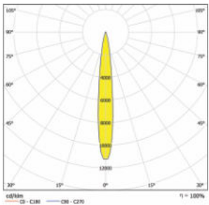
BO177-Sunbeam-1x1-3535-10°
