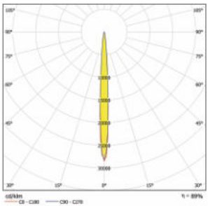
BO201-Sunbeam-1x1-3535-7°
