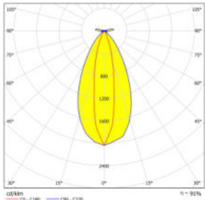
BO173-Sunbeam-1x1-3535-15x45°
