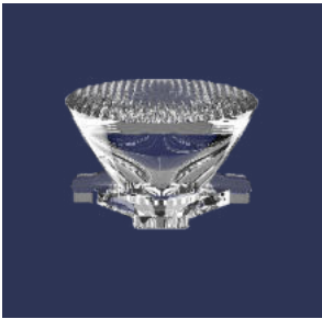
BO202-Sunbeam-1x1-3535-15x45°
