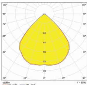
BO119-Custom-18x1-5050-90°
