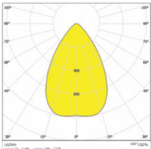
BO39-Sunbeam-1x1-3030-45°
