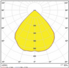
BO135-Aura-5050-90°(3 Rings)
