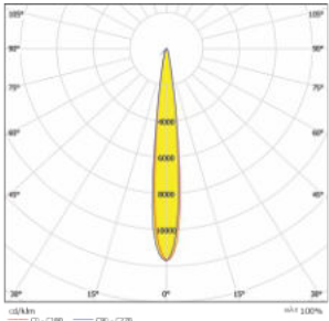
BO172-Sunbeam-1x1-3535 -17°
