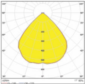
BO194-Aura-2835-3030-90° (4 Rings)
