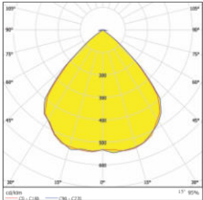
BO11-Shimmer-16x1-2835/3030-90°
